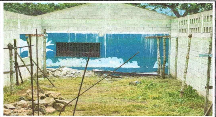
Foto 2: Rehabilitación de Estructura de techo a estructura de costaneras, láminas troqueladas y piso de torta de concreto.
