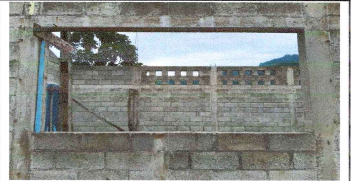
Foto 6: Rehabilitación de ventanas a ventana balcon con vidrios y cernido de paredes interior y exterior.
